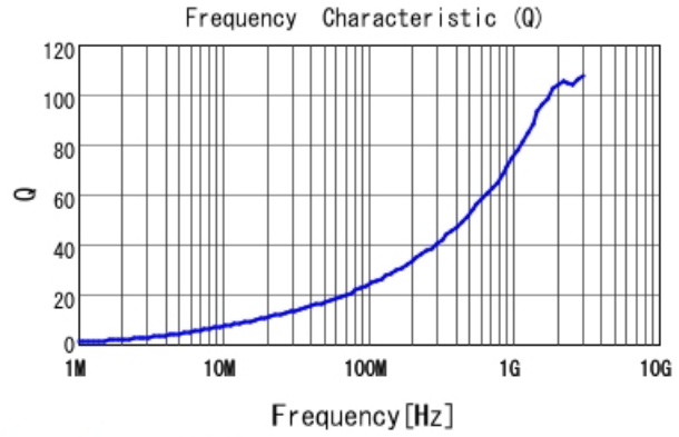
LQW15AN7N0G8Z Q
