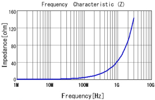
LQW15AN7N0G8Z |Z|
