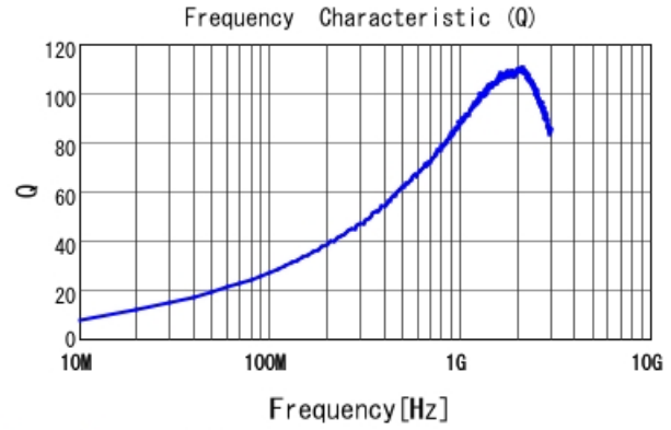
LQW18AN10NJ00 Q
