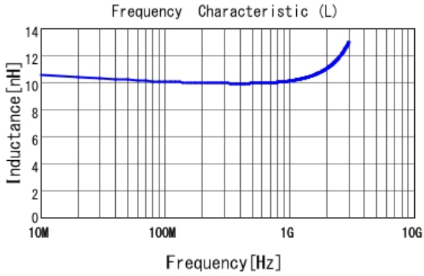
LQW18AN10NJ00 L
