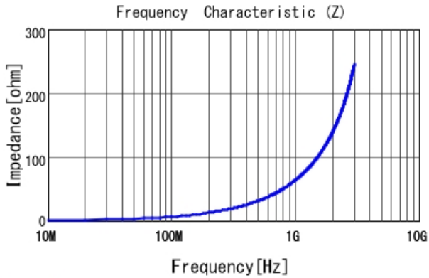
LQW18AN10NJ00 |Z|
