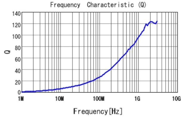
LQW15AN4N1B80 Q
