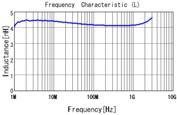
LQW15AN4N1B80 L
