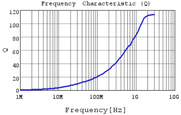
LQW15AN3N0B8Z Q
