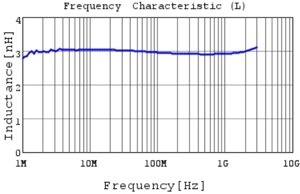
LQW15AN3N0B8Z L
