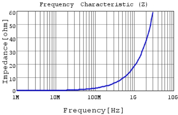
LQW15AN3N0B8Z |Z|
