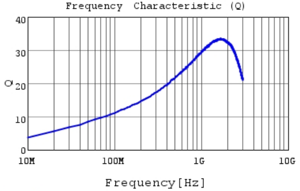
LQG15HS8N2G02 Q
