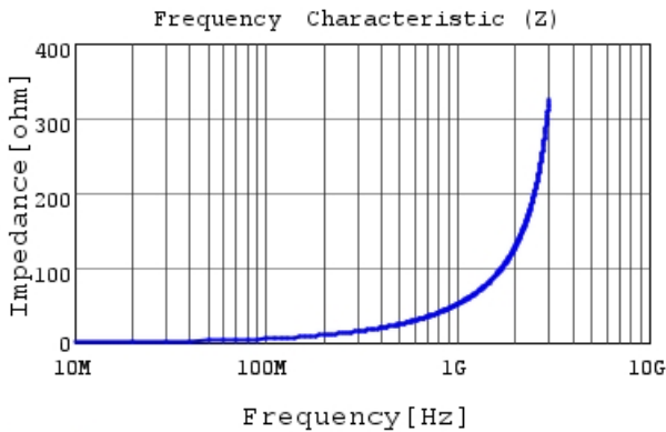
LQG15HS8N2G02 |Z|
