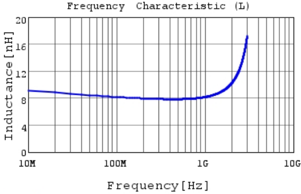
LQG15HS8N2G02 L
