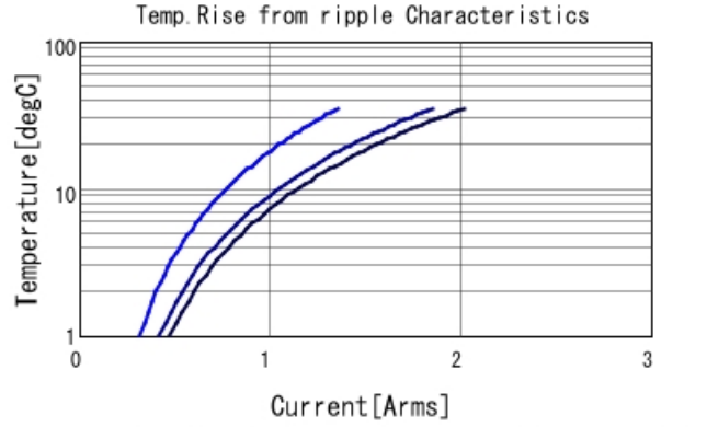
GCM188R71E154KA37 Temp. rise — 400kHz — 800
