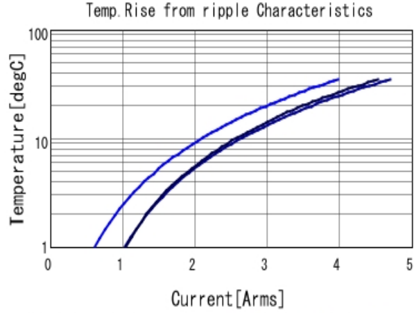
GRJ31CR70J226KE12 Temp. rise ■ 80kHz ■ 400kHz ■ 800kHz
