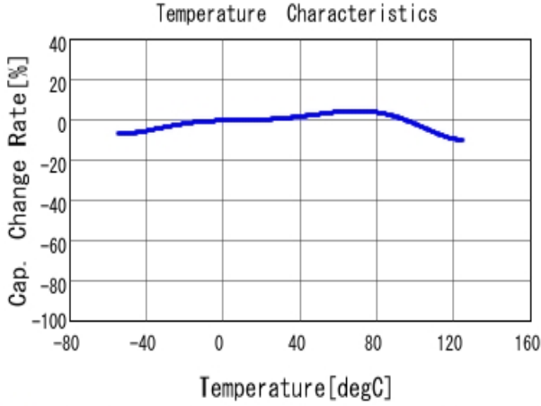
■ GRJ31CR70J226KE12 C-Temp. capchange, DCO. 0V, ACO. 5Vrm
