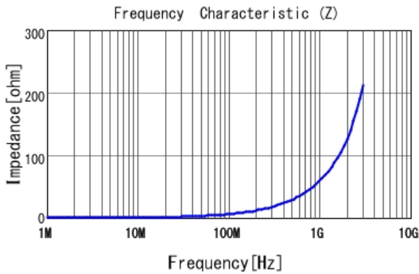
LQW15AN9N5G8Z |Z|
