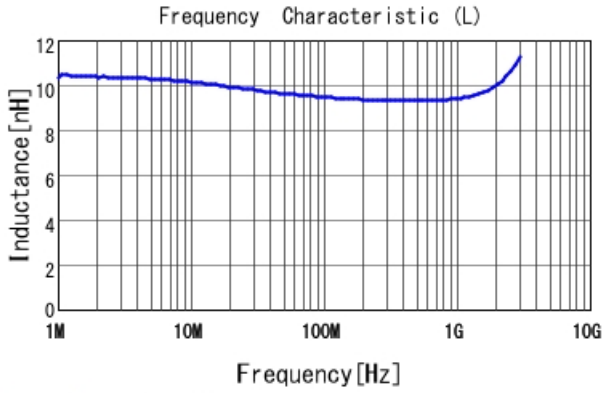
LQW15AN9N5G8Z L
