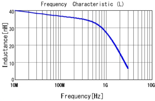
LQW15CA39NK00 L
