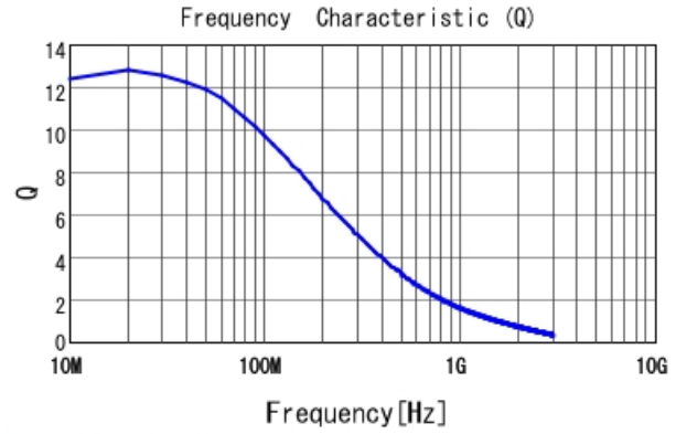
LQW15CA39NK00 Q
