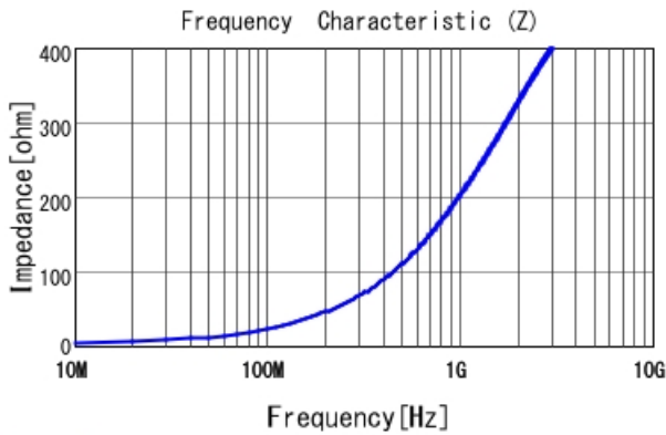
LQW15CA39NK00 |Z|
