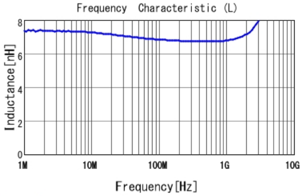
LQW15AN6N8J80 L
