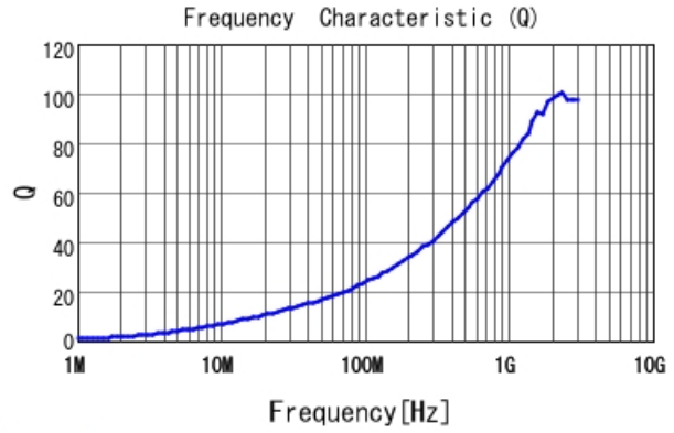
LQW15AN6N8J80 Q
