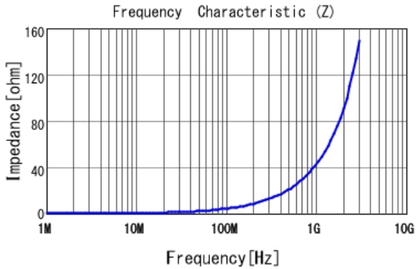
LQW15AN6N8J80 |Z|
