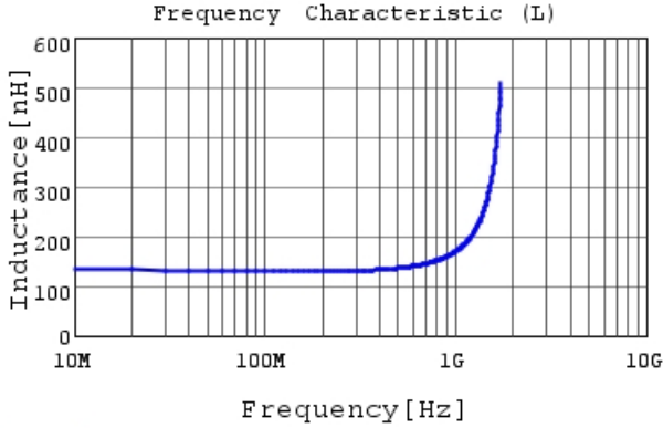
LQW18ANR13G00 L
