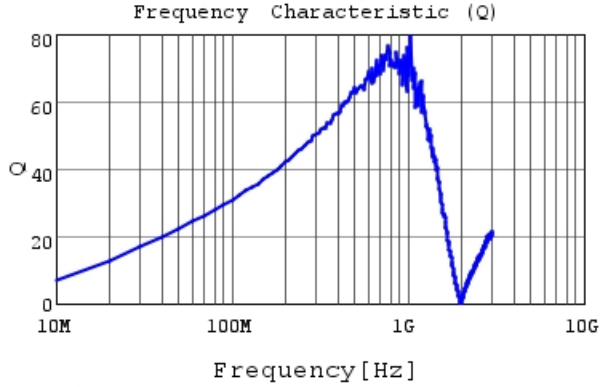
LQW18ANR13G00 Q
