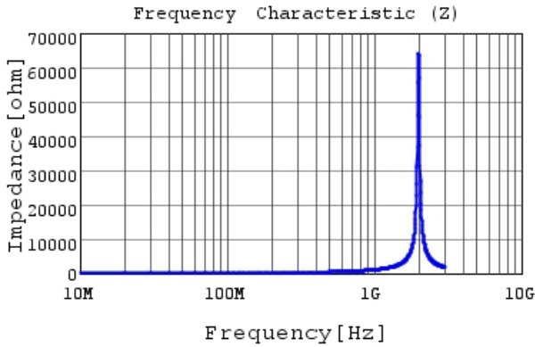
LQW18ANR13G00 |Z|
