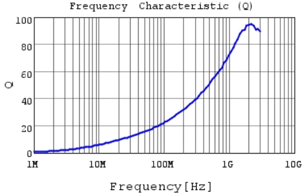
LQW15AN6N6G80 Q
