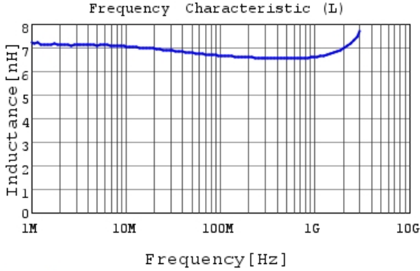
LQW15AN6N6G80 L
