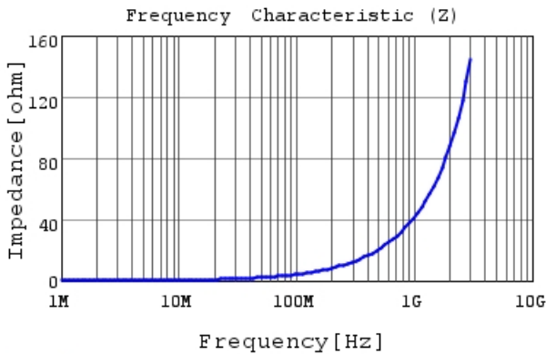
LQW15AN6N6G80 |Z|
