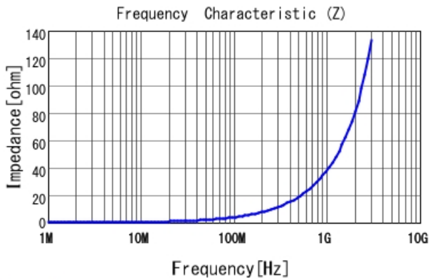
LQW15AN6N2G80 |Z|
