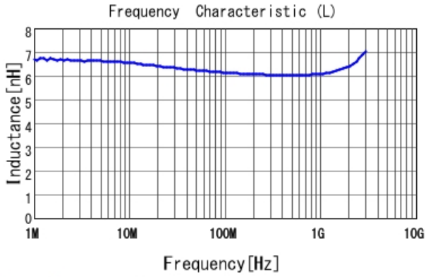
LQW15AN6N2G80 L
