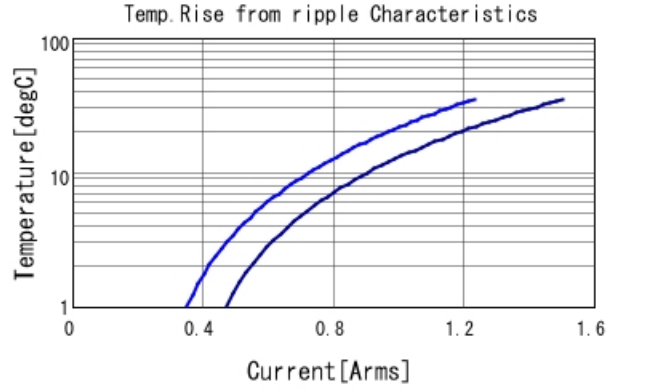
GRM152R60J104ME19 Temp. rise — 500kHz — 1MHz
