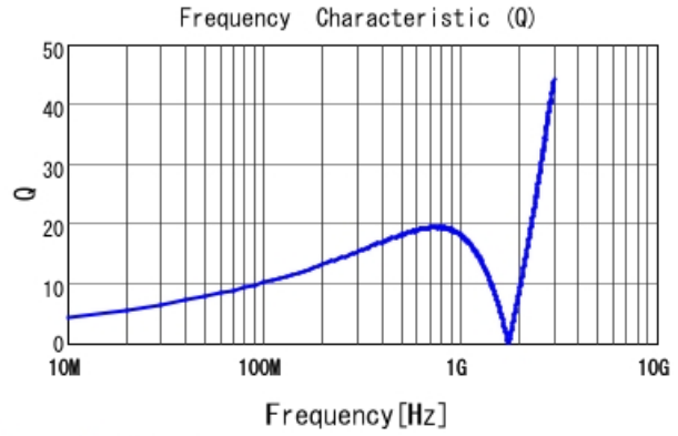
LQG15HZ39NH02 Q
