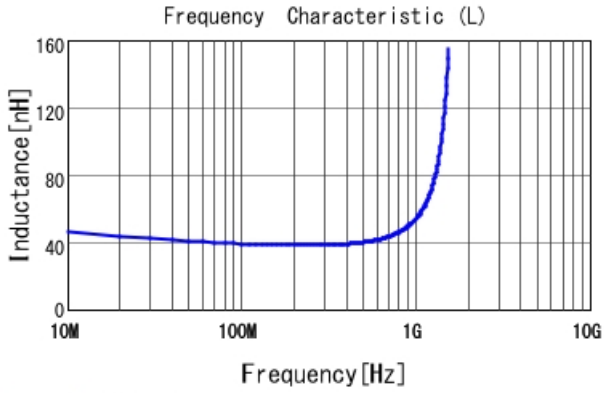
LQG15HZ39NH02 L
