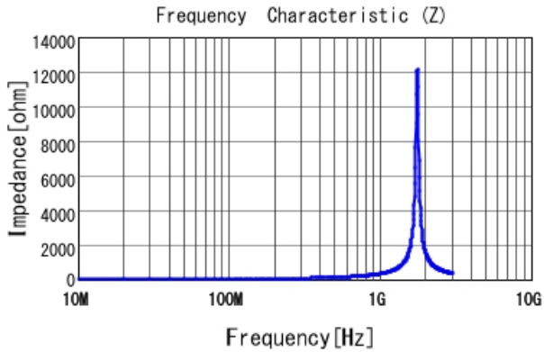
LQG15HZ39NH02 |Z|
