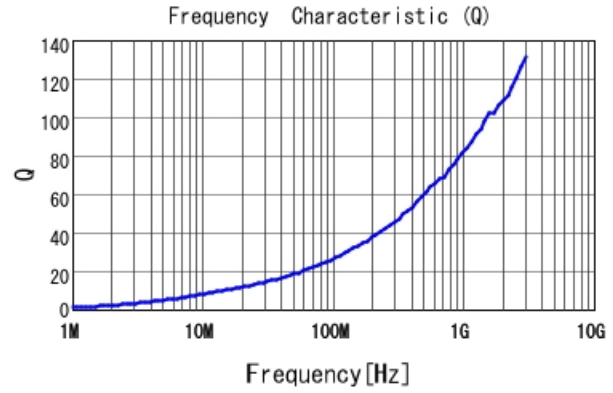
LQW15AN3N7G80 Q
