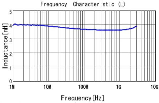
LQW15AN3N7G80 L
