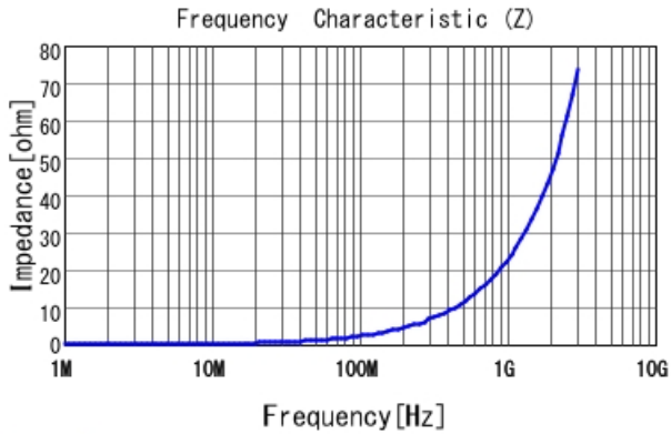
LQW15AN3N7G80 |Z|
