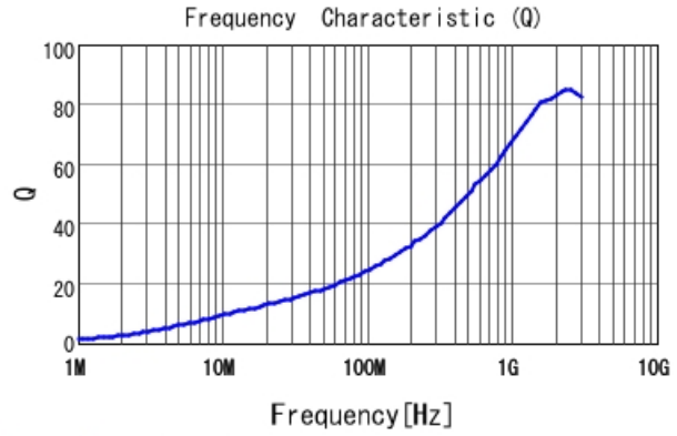
LQW15AN8N9G80 Q
