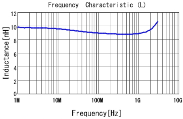
LQW15AN8N9G80 L
