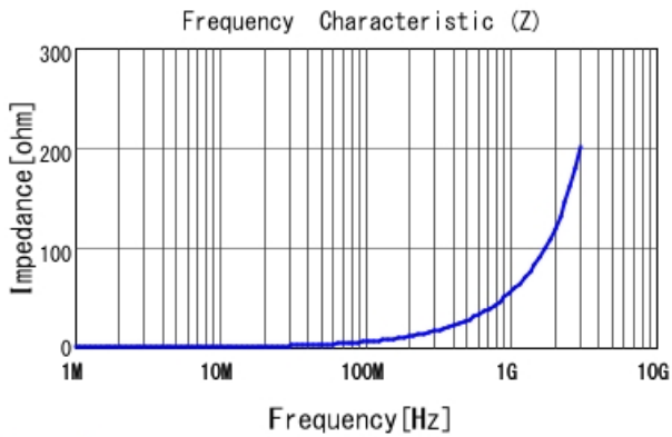
LQW15AN8N9G80 |Z|
