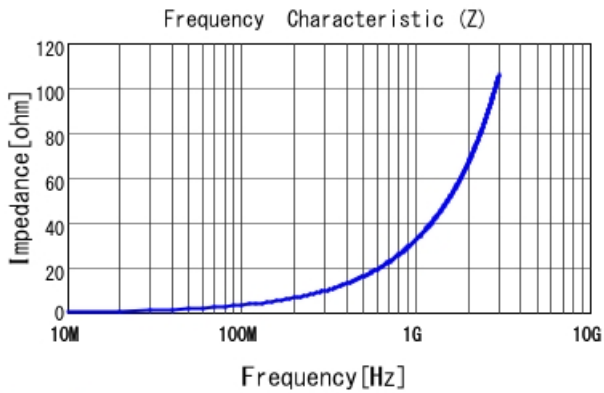
LQW15AN5N1D10 |Z|
