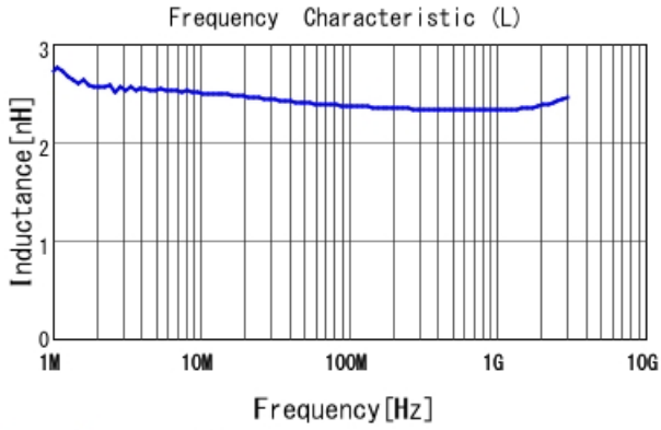
LQW15AN2N4C80 L
