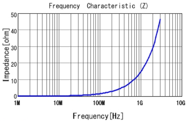
LQW15AN2N4C80 |Z|
