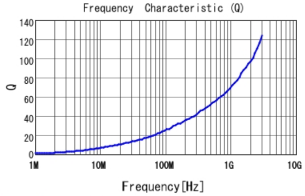
LQW15AN2N4C80 Q
