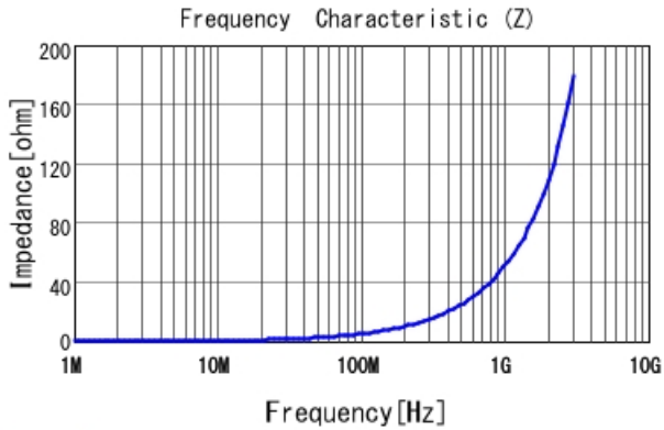
LQW18AN8N2G80 |Z|
