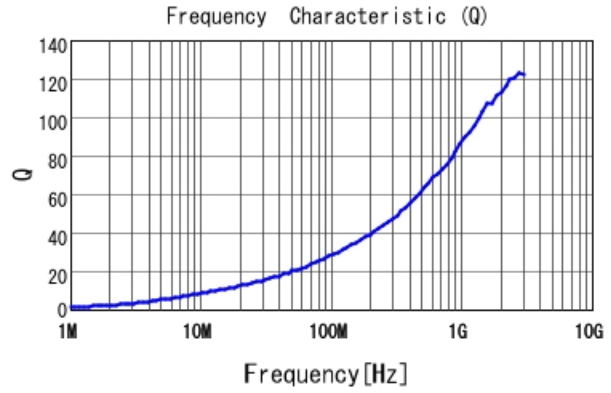
LQW18AN8N2G80 Q
