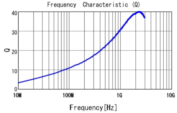
LQG15HH5N1S02 Q
