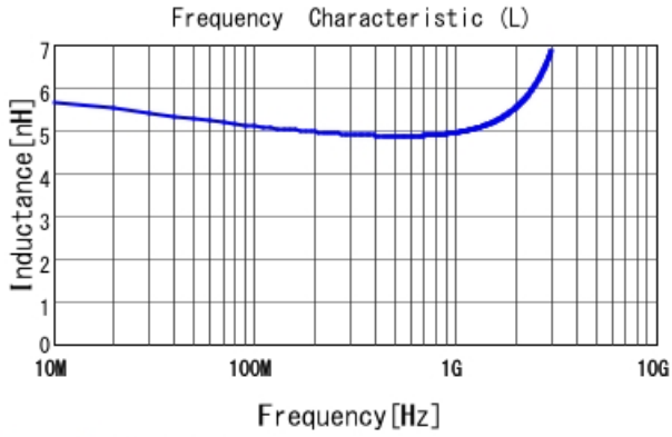
LQG15HH5N1S02 L
