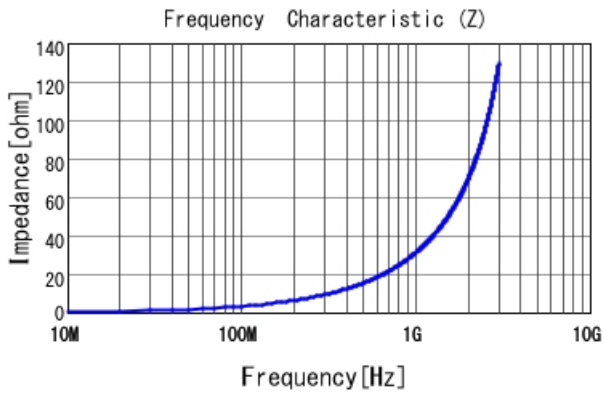
LQG15HH5N1S02 |Z|
