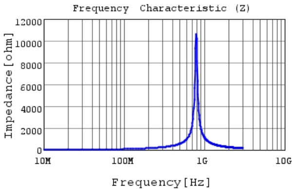
LQG15HSR12H02 |Z|
