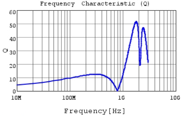
LQG15HSR12H02 Q
