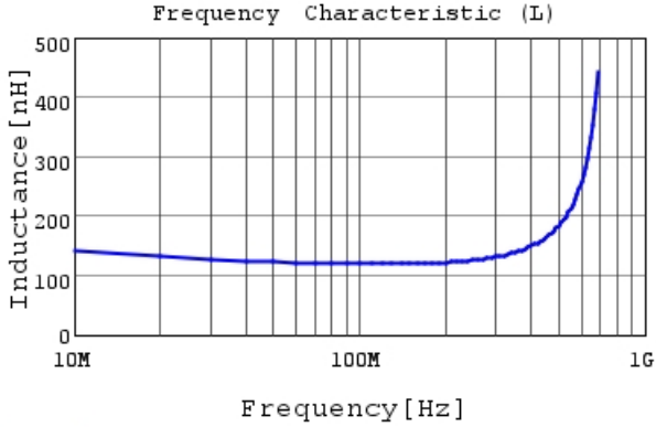
LQG15HSR12H02 L
