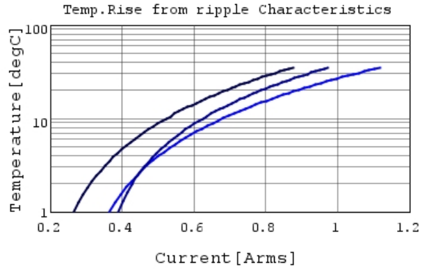
GJM0335C1E100JB01 Temp.rise 1GHz 2
