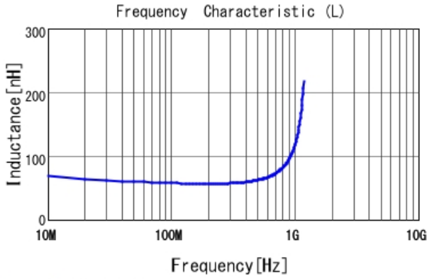
LQG15HH56NG02 L
