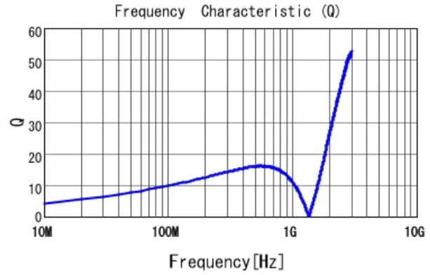
LQG15HH56NG02 Q
