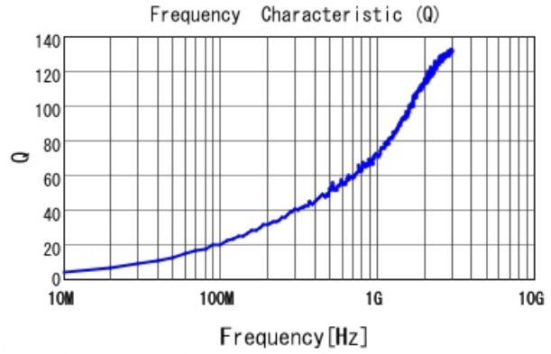
LQW15AN1N3D10 Q
