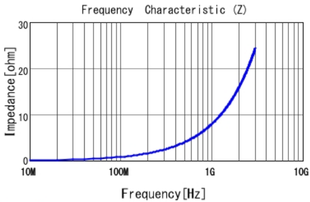
LQW15AN1N3D10 |Z|
