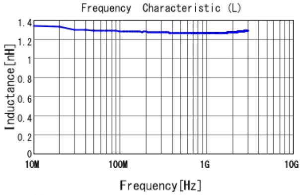
LQW15AN1N3D10 L
