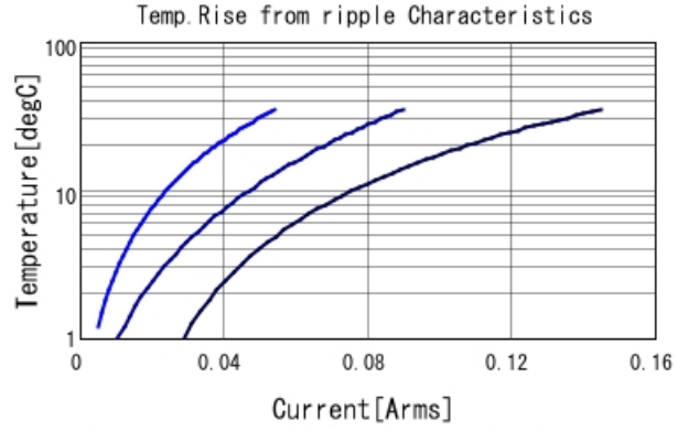
GRM21AR72E222KW01 Temp. rise — 30kHz — 100kHz
