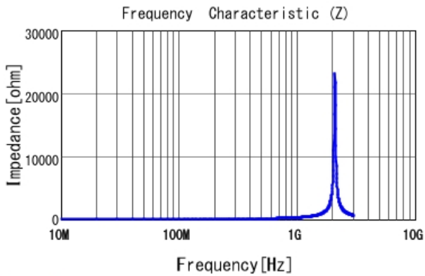
LQG15WH39NJ02 |Z|
