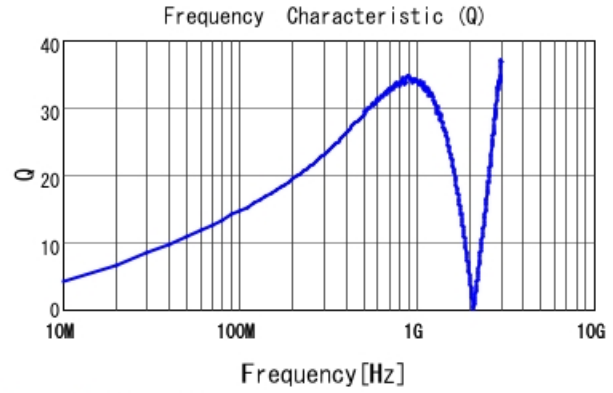
LQG15WH39NJ02 Q
