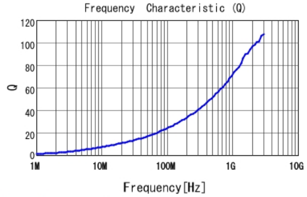
LQW15AN5N6G8Z Q
