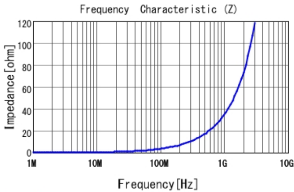
LQW15AN5N6G8Z |Z|
