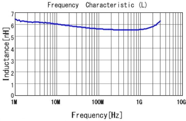
LQW15AN5N6G8Z L
