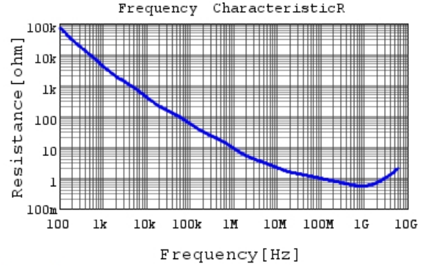
GRM033B11E221KA01 R DCOV, 20degC
