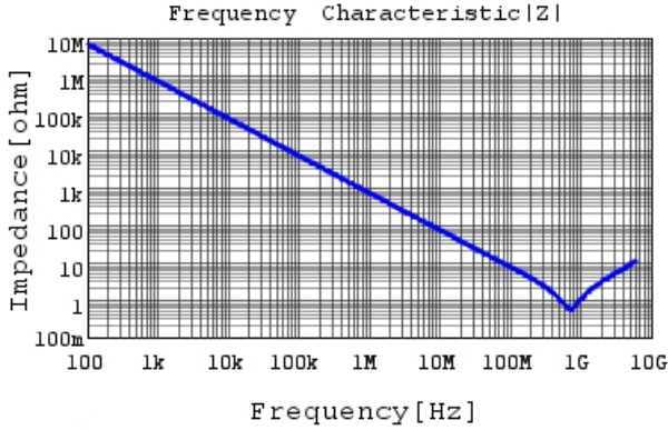
GRM033B11E221KA01 |Z| DCOV, 20degC
