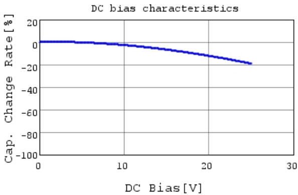
GRM033B11E221KA01 C-DC bias capchange, 20.0c
