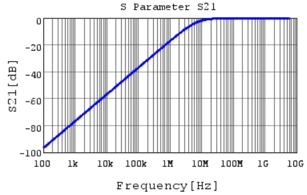
GRM033B11E221KA01 S21 DC0V, 20degC
