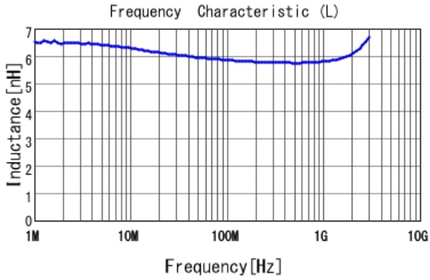
LQW15AN5N9C8Z L
