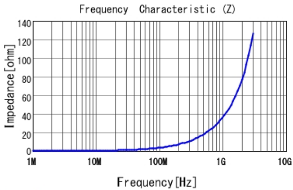
LQW15AN5N9C8Z |Z|
