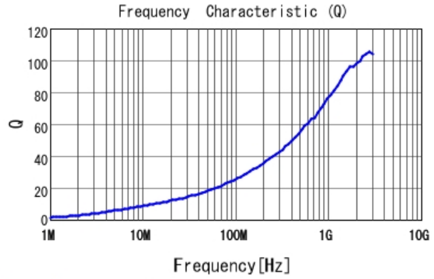
LQW15AN5N9C8Z Q
