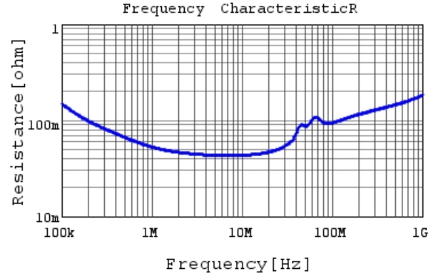
RDER71H104K0S1H03A R DC0V, 25degC
