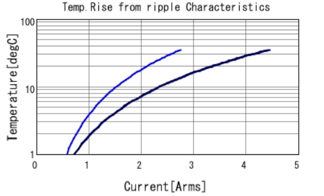
GRM31MR71E225KA93 Temp. rise — 100kHz — 500
