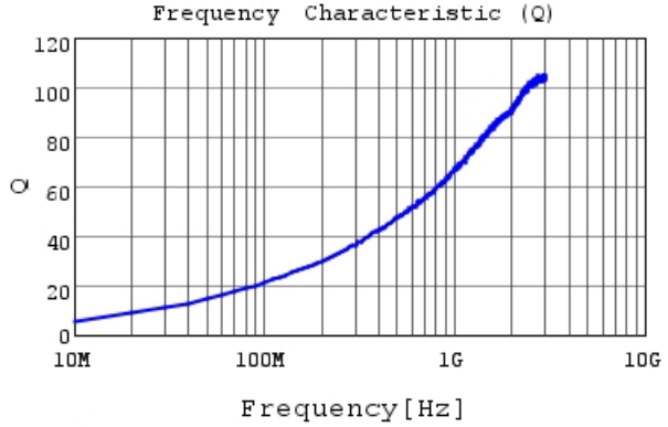
LQW15AN6N8G00 Q
