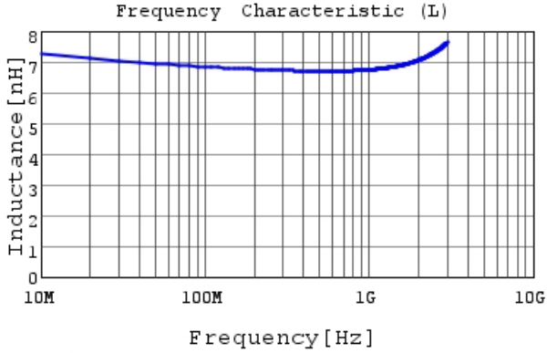
LQW15AN6N8G00 L
