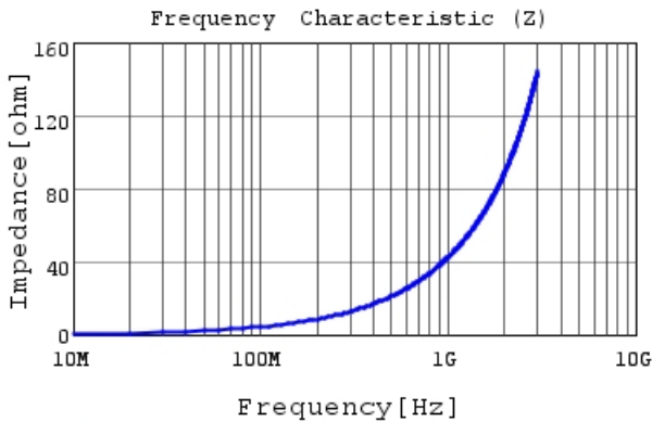
LQW15AN6N8G00 |Z|
