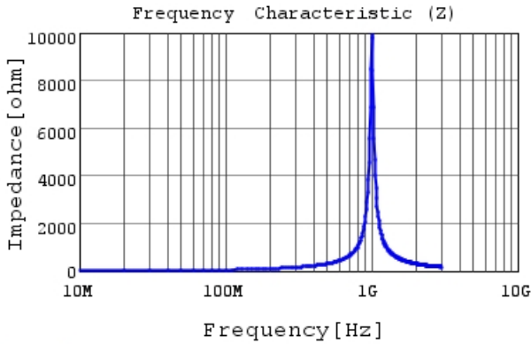
LQG15HS82NH02 |Z|
