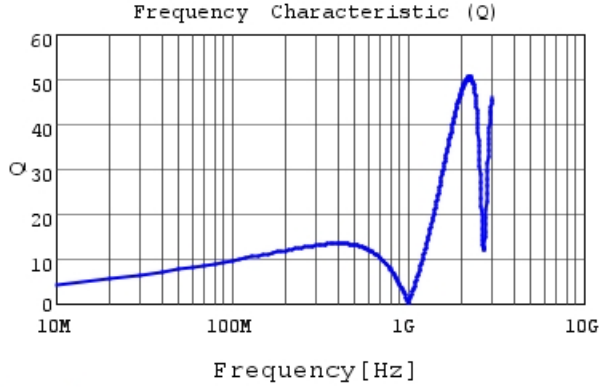
LQG15HS82NH02 Q
