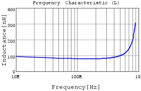
LQG15HS82NH02 L
