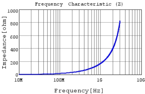
LQW15AN27NG00 |Z|
