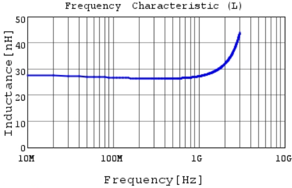
LQW15AN27NG00 L
