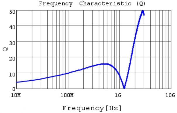
LQG15HN68NJ02 Q
