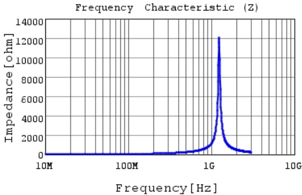
LQG15HN68NJ02 |Z|
