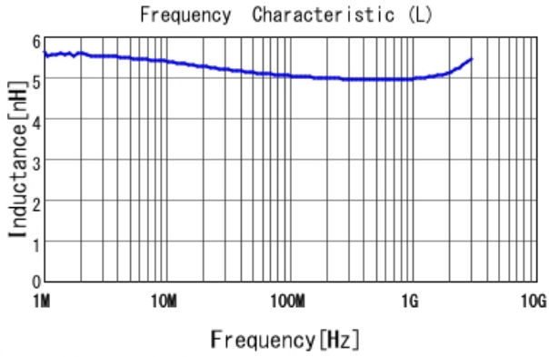
LQW15AN5N0C80 L
