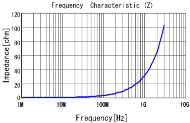
LQW15AN5N0C80 |Z|
