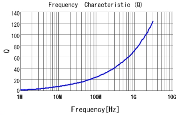
LQW15AN5N0C80 Q
