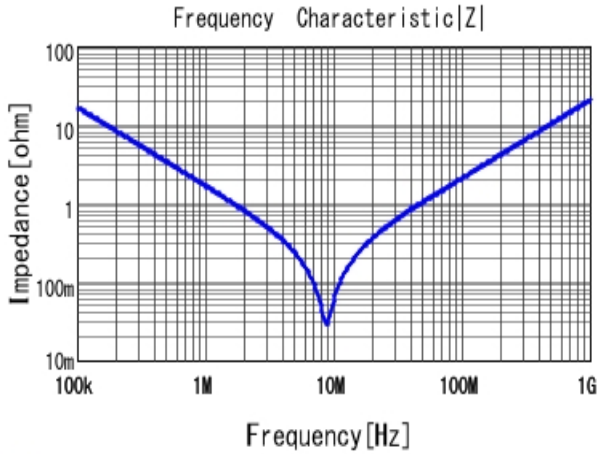
■ RCER71H104K0DBH03A |Z| DC0V, 25degC
