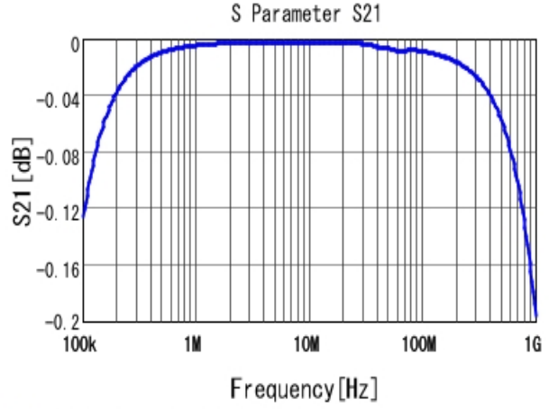
■ RCER71H104K0DBH03A S21 DC0V, 25degC
