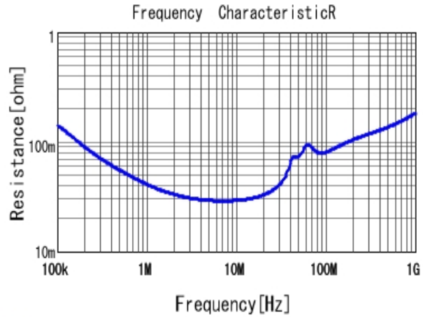
■ RCER71H104K0DBH03A R DC0V, 25degC
