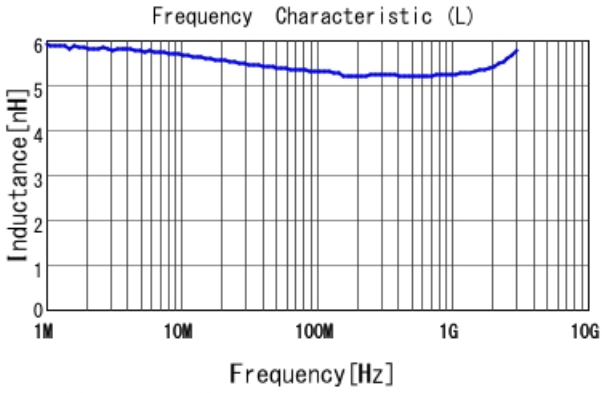
LQW15AN5N3B8Z L
