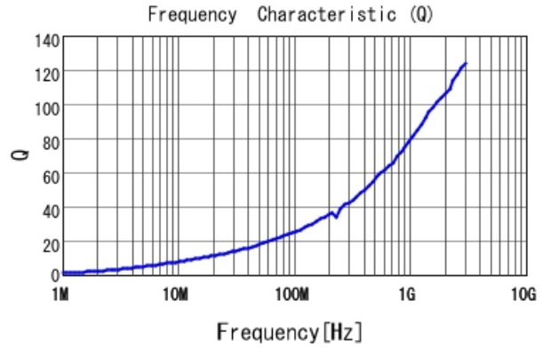
LQW15AN5N3B8Z Q
