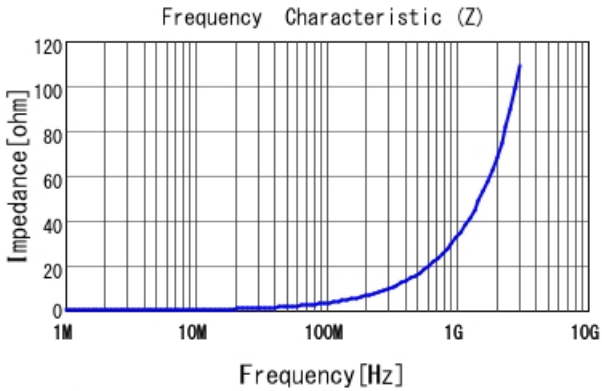
LQW15AN5N3B8Z |Z|
