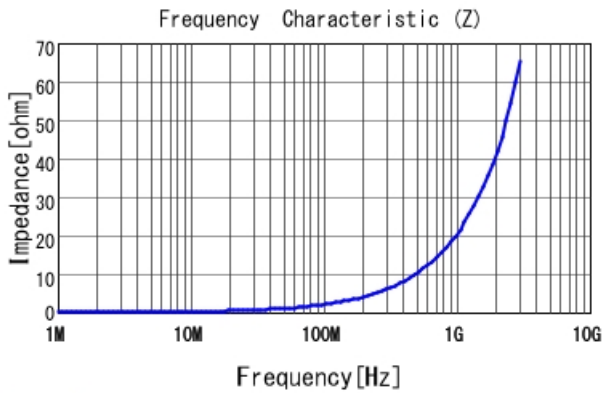
LQW15AN3N3B80 |Z|
