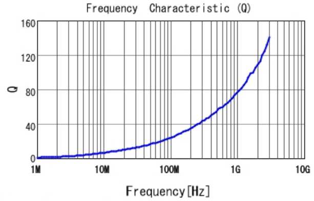
LQW15AN3N3B80 Q
