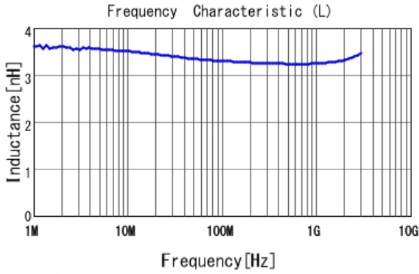
LQW15AN3N3B80 L
