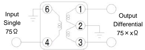
2) #458PT-1720 (Impedance Ratio=75Ω:50Ω)
