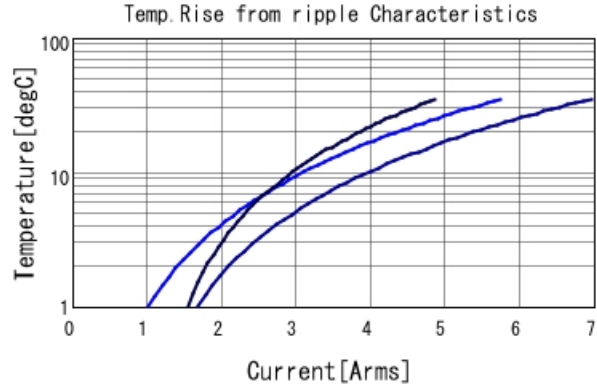
GRM32ER61E226KE15 Temp. rise — 80kHz — 400kHz
