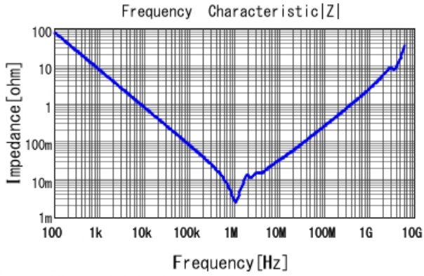
GRM32ER61E226KE15 |Z| DCOV, 25degC
