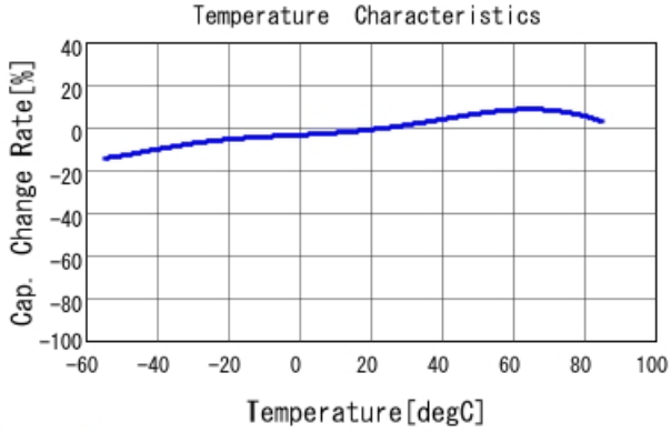
GRM32ER61E226KE15 C-Temp. capchange, DCO. 0V, ACO. 5
