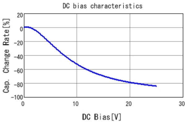
GRM32ER61E226KE15 C-DC bias capchange, 25.0degC, A
