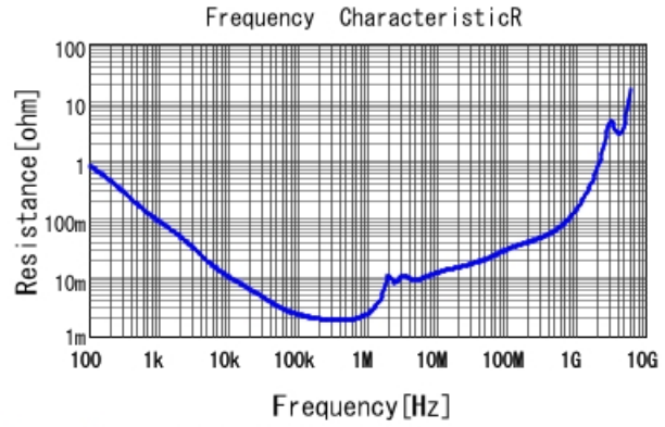
GRM32ER61E226KE15 R DCOV, 25degC
