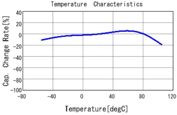
■ GRM32EC81C476ME15 C-Temp. capchange, DCO. 0V, ACO. 5Vrm
