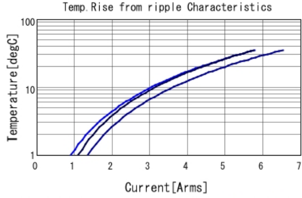
GRM32EC81C476ME15 Temp. rise ■ 60kHz ■ 300kHz ■ 600kHz
