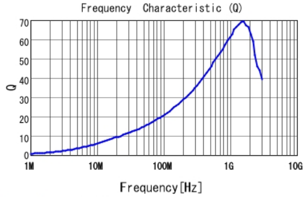
LQW15AN24NG8Z Q
