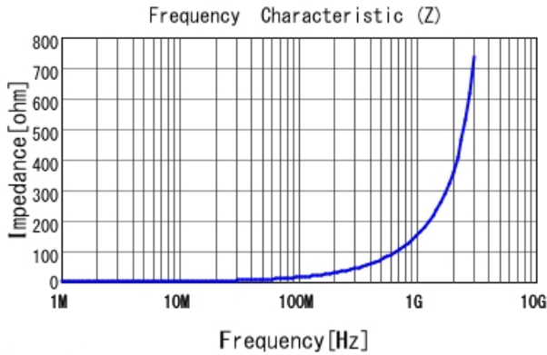
LQW15AN24NG8Z |Z|
