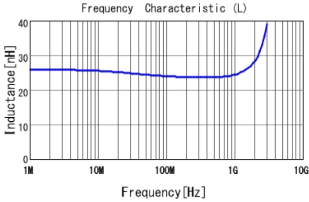
LQW15AN24NG8Z L
