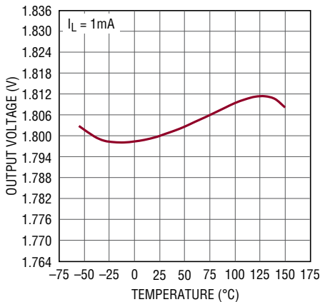
LT3065-1.8 Output Voltage
