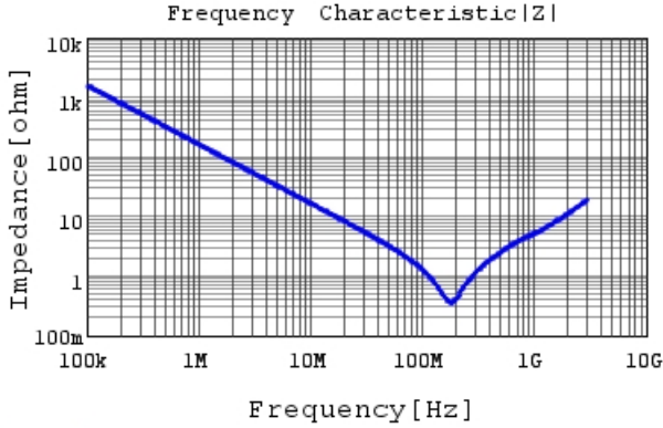
GCJ31BR73A102KXJ1 |Z| DC0V, 25degC
