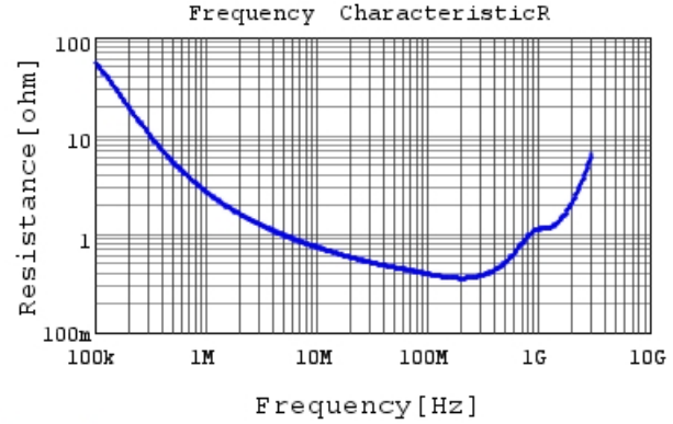
GCJ31BR73A102KXJ1 R DC0V, 25degC
