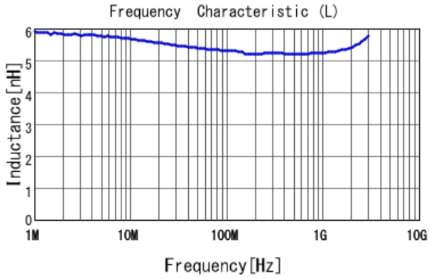
LQW15AN5N3B80 L
