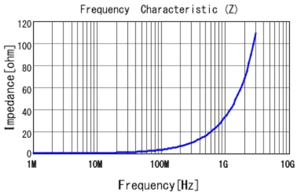
LQW15AN5N3B80 |Z|
