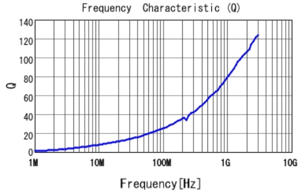
LQW15AN5N3B80 Q
