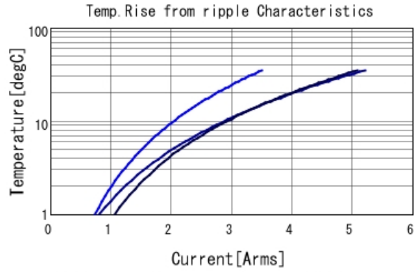
GRM43ER71H225KA01 Temp. rise — 100kHz — 500
