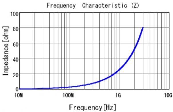
LQW15AN4N1B0Z |Z|
