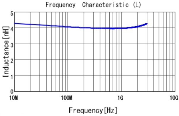
LQW15AN4N1B0Z L
