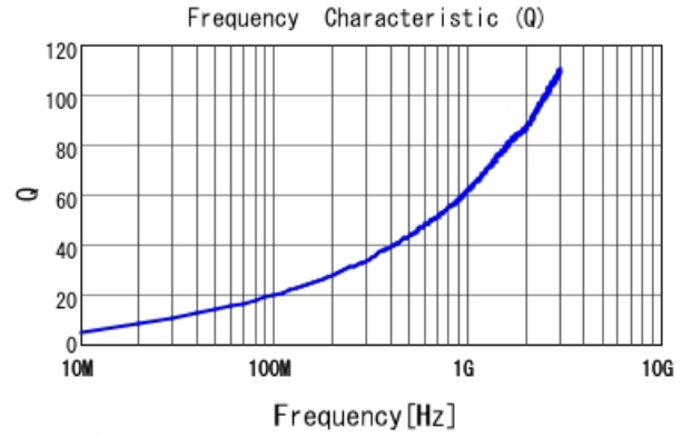
LQW15AN4N1B0Z Q
