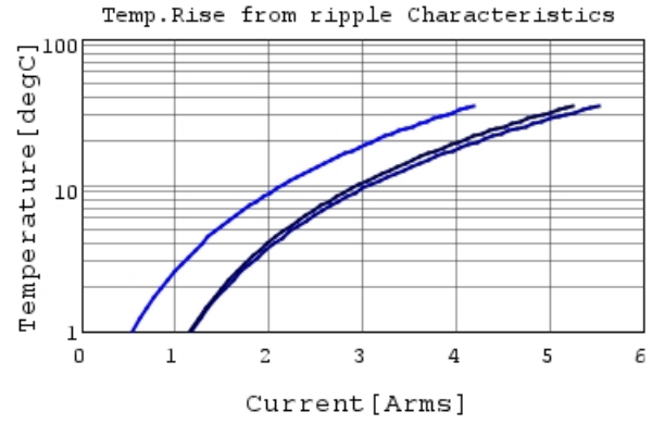
GRT21BC71E106KE13 Temp.rise — 80kHz
